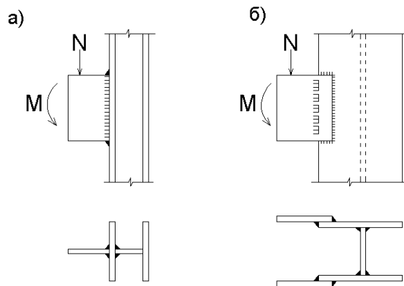
а — перпендикулярной; б — параллельной плоскости расположения швов Рисунок 10.2 — Расположение сварных соединений с угловыми швами при действии момента в плоскости
