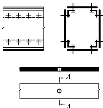
Рисунок В.1 – Расположение проверяемого на выносливость расчетного сечения А–А по основному металлу в сечениях нетто по соединительным болтам составных элементов, а также у свободного отверстия
