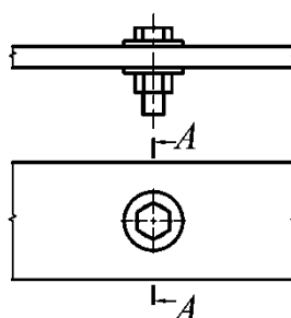
Рисунок В.2 – Расположение проверяемого на выносливость расчетного сечения А–А по основному металлу в сечениях нетто у отверстия с поставленным в него высокопрочным болтом, затянутым на нормативное усилие
