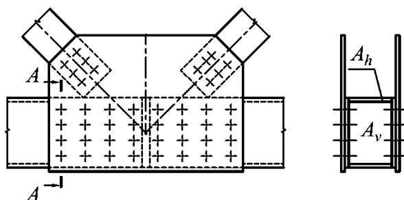
Рисунок В.5 – Расположение проверяемого на выносливость расчетного сечения А–А по основному металлу в сечении брутто по первому ряду высокопрочных болтов в креплении к узлу или в стыке двухстенчатых элементов с односторонними накладками
