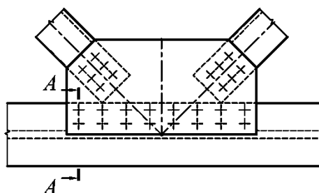
Рисунок В.3 – Расположение проверяемого на выносливость расчетного сечения А–А по основному металлу в сечении брутто по первому ряду высокопрочных болтов в прикреплении фасонки к нестыкуемым в данном узле поясам сплошных балок и элементам решетчатых форм
