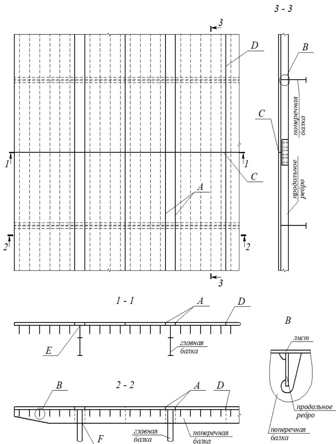
Рисунок Д.1 – Расположение зон ортотропной плиты, рассчитываемых на выносливость.
