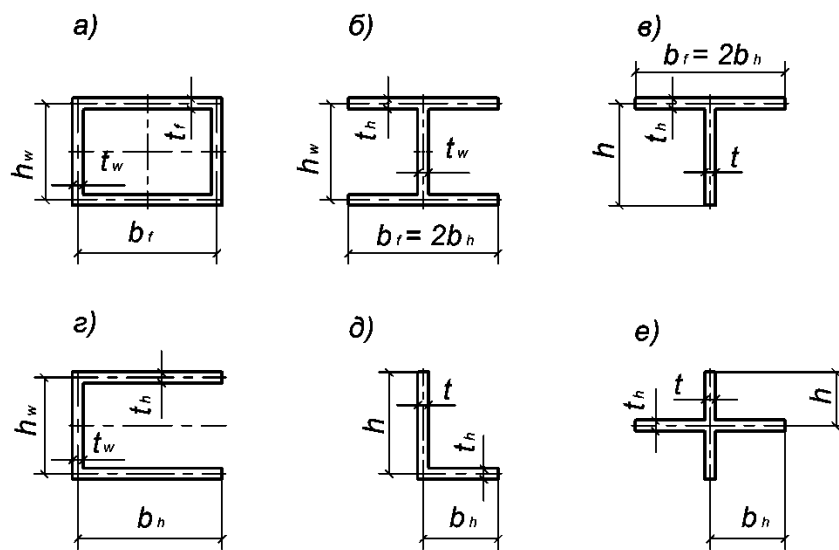
Рисунок 9.3.3.1 — Схемы расчетных сечений элементов, не подкрепленных ребрами жесткости
