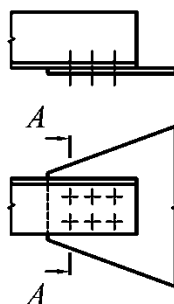
Рисунок В.6 – Расположение проверяемого на выносливость расчетного сечения А–А по основному металлу в сечении брутто по первому ряду высокопрочных болтов в креплении к узлу или в стыке одностенчатых элементов с односторонними накладками
