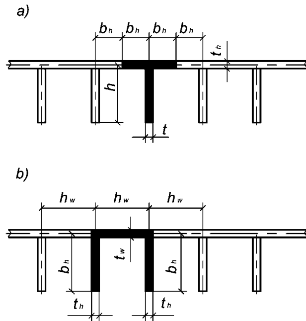
Рисунок 9.3.4.1 — Схемы расчетных сечений пластинок ортотропных плит. Расчетные длины
