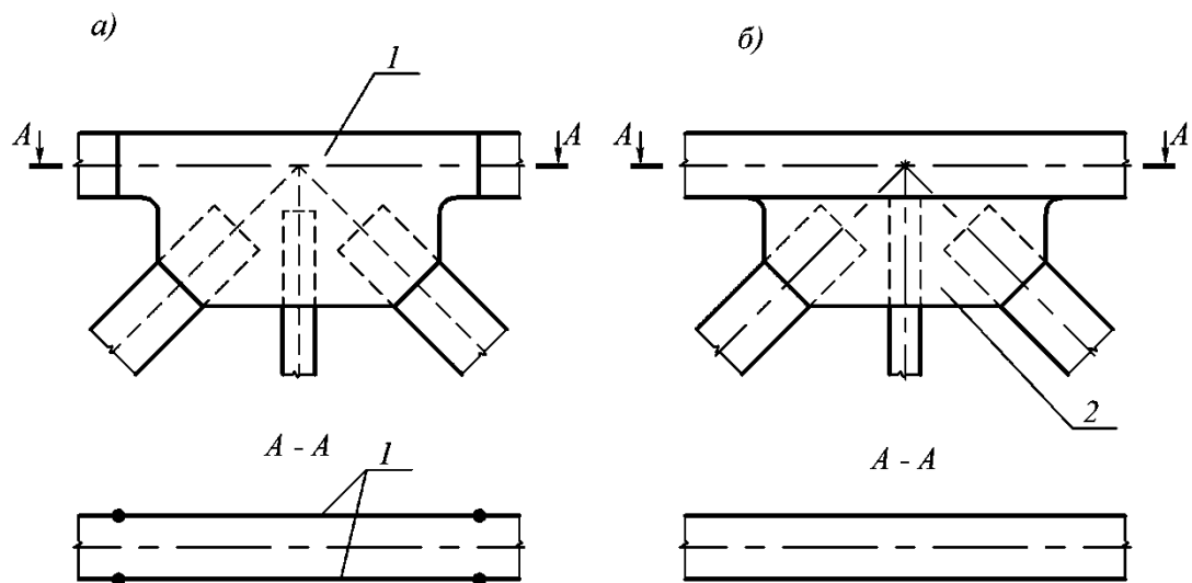
а — с фасонками - вставками; б — с фасонками – приставками; 1 – фасонка – вставка; 2 – фасонка - приставка
